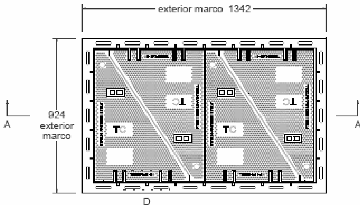
vista en planta 1:20
