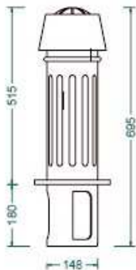
vista alzado 1:10
