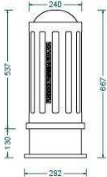
vista alzado 1:10
